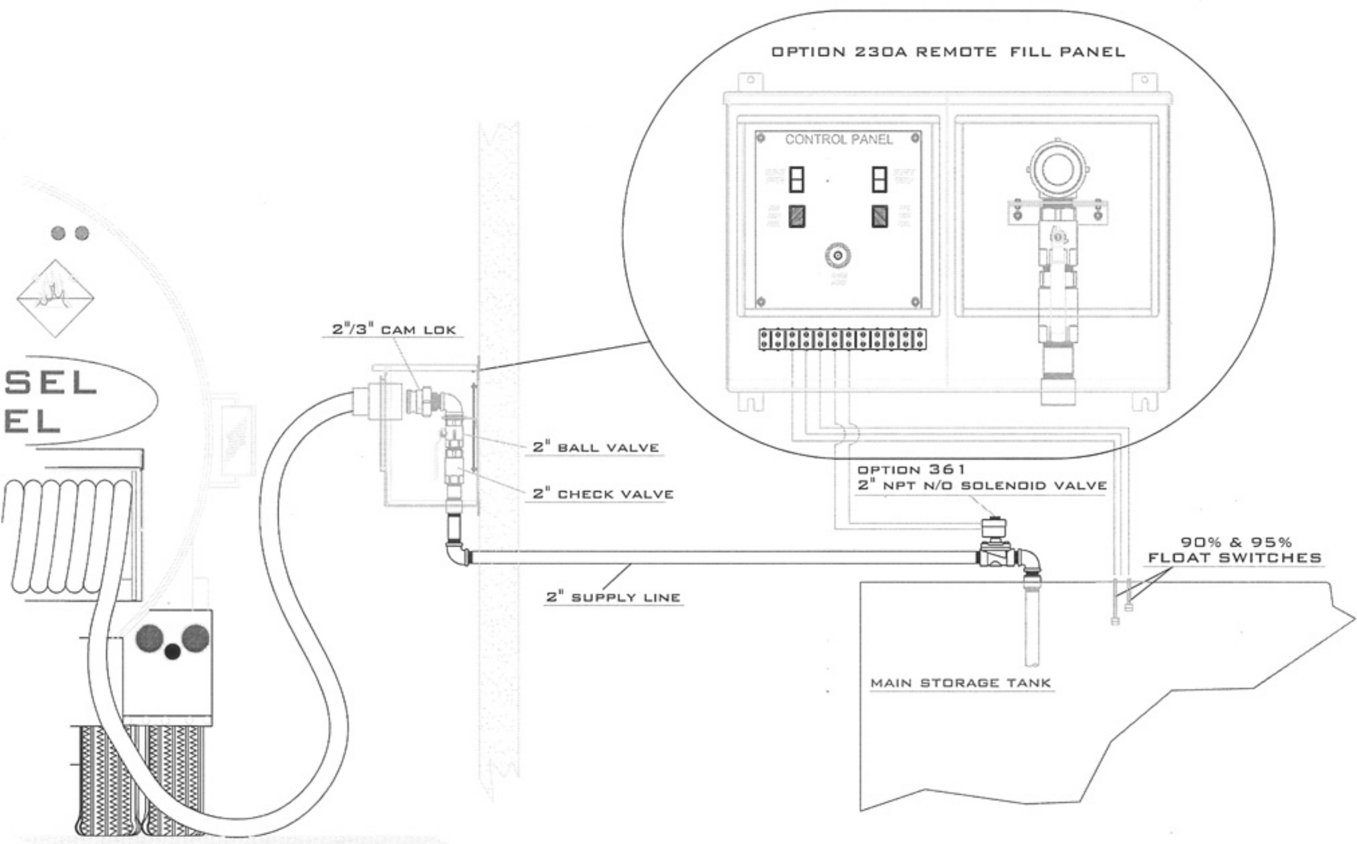
230A_REMOTE_FILL_LAYOUT
